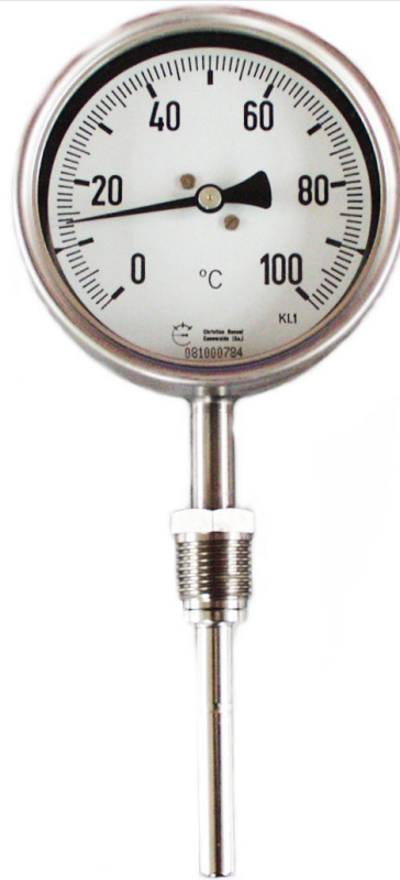
Gasdruck-Thermometer mit starrem Fühler Industrieausführung
